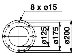
Насос с фланцем Grundfos
