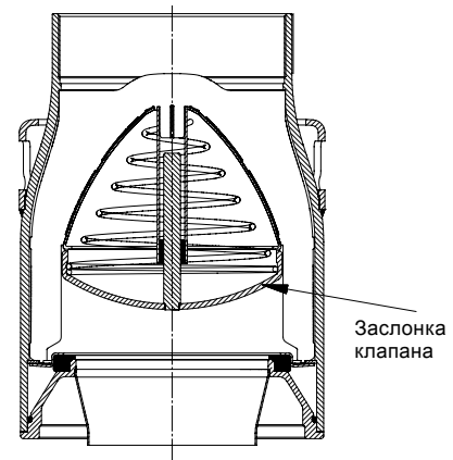
Рис. 5 Обратный клапан
